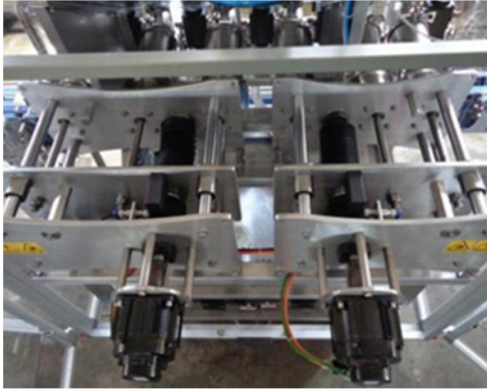
YASKAWA Particolare gruppo BRUSHLESS MOTOMAN ROBOTICS
